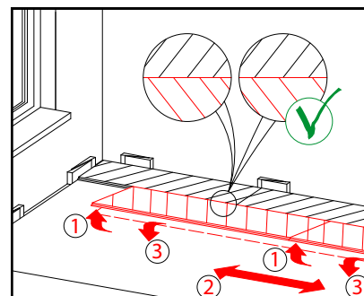
3. Ausrichtung Riegelversatz:
